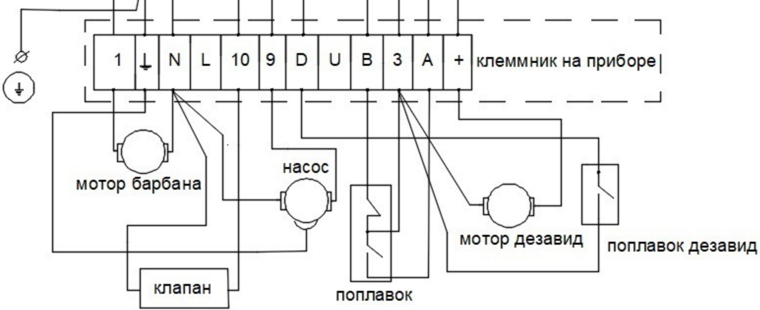
СХЕМА ЭЛЕКТРИЧЕСКАЯ МОНТАЖНАЯ FANLINE PRO-4005K-4805K-6005K
