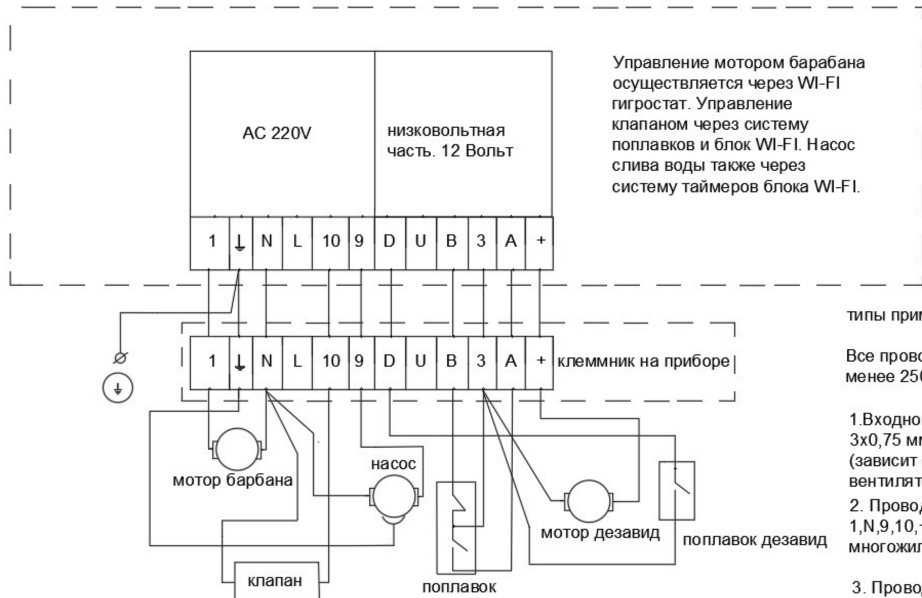
СХЕМА ЭЛЕКТРИЧЕСКАЯ МОНТАЖНАЯ FANLINE PRO-4005K-4805K Wi-Fi
