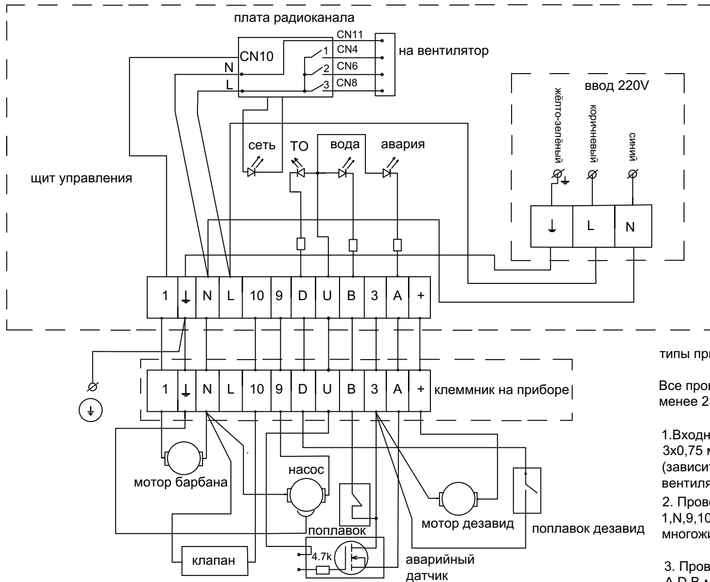
СХЕМА ЭЛЕКТРИЧЕСКАЯ МОНТАЖНАЯ FANLINE PRO-4005K-4805K
